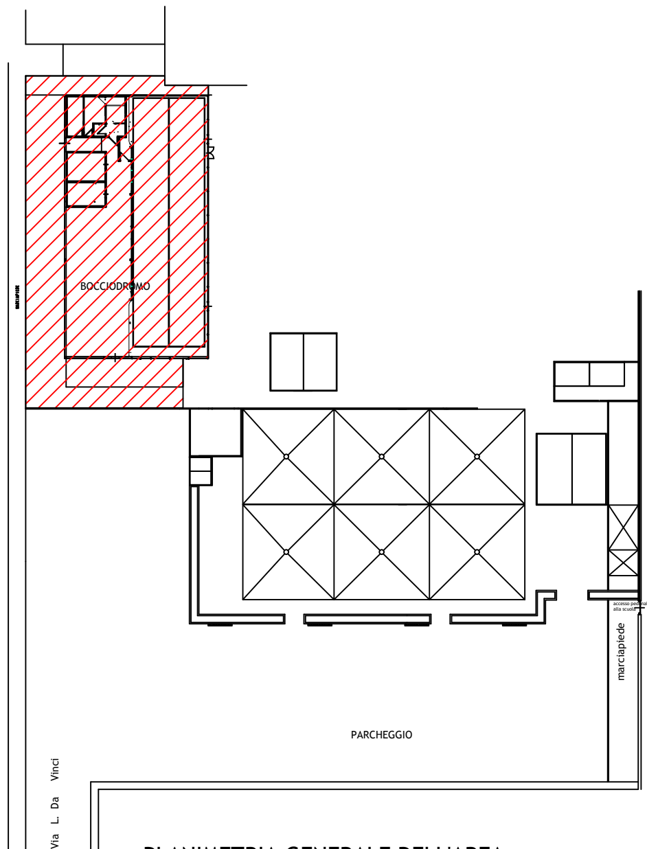
PLANIMETRIA GENERALE DELL'AREA SCALA 1/500
